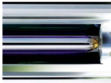
Bild 7: Exklusive UV Trocknung, vollständig gekapselt, Ozonfrei, ohne Abluft und geräuschlos
